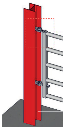
Poteau de charpente H
