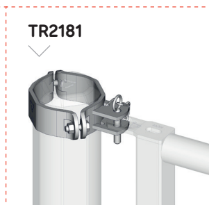
Poteau TRÈFLE Ø 140 mm
